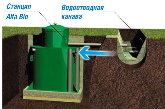
Вид 3. Контруклон
